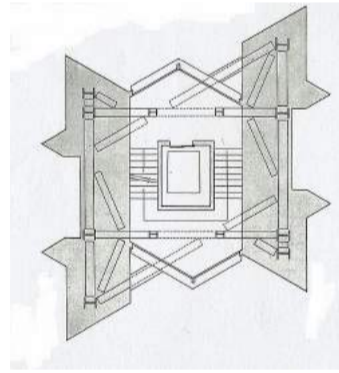
図3：百年記念塔の水平断面図(9～24階)
